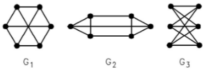
Рисунок 1 – Графы сети
