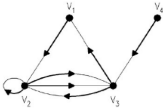
Рисунок 1 – Граф сети
